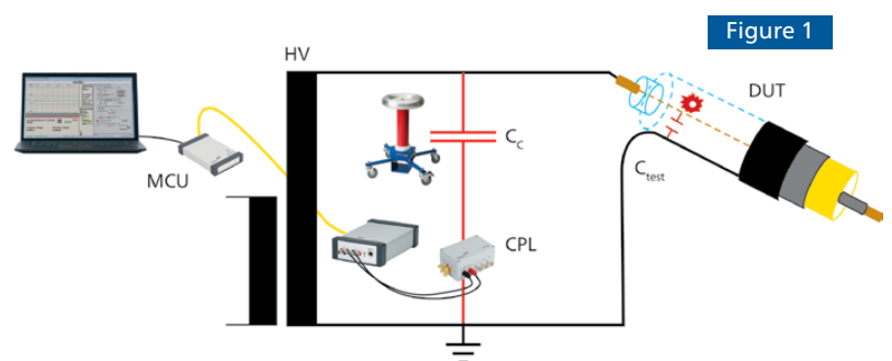
Figure 1 Montage de mesure de DP type conformément à la norme CEI 60270
