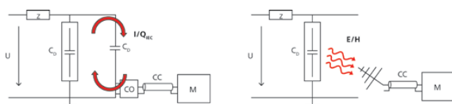
Mesure des DP conforme à la norme CEI
