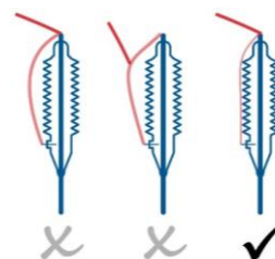
Figura 8: Configuración recomendada según la norma IEC 60076-18
