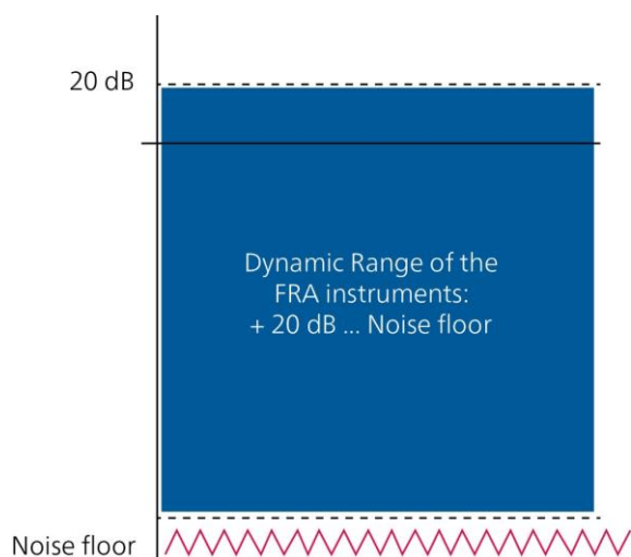
Figura 5: Ilustración del suelo de ruido y el rango dinámico
