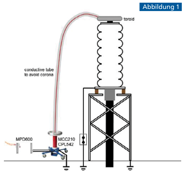
Basisschaltbild eines Koppelkondensators an einem Kabelendverschluss
