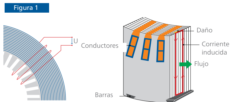
Figura 1 Lado izquierdo: Devanado auxiliar con indicación de líneas de flujo azules; Lado derecho: mayor corriente parásita debido a un núcleo del estator dañado.
