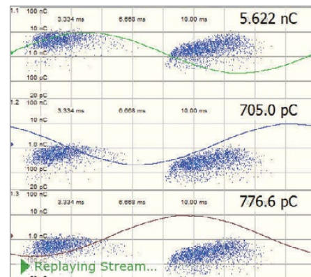
Fuente de DP separada
