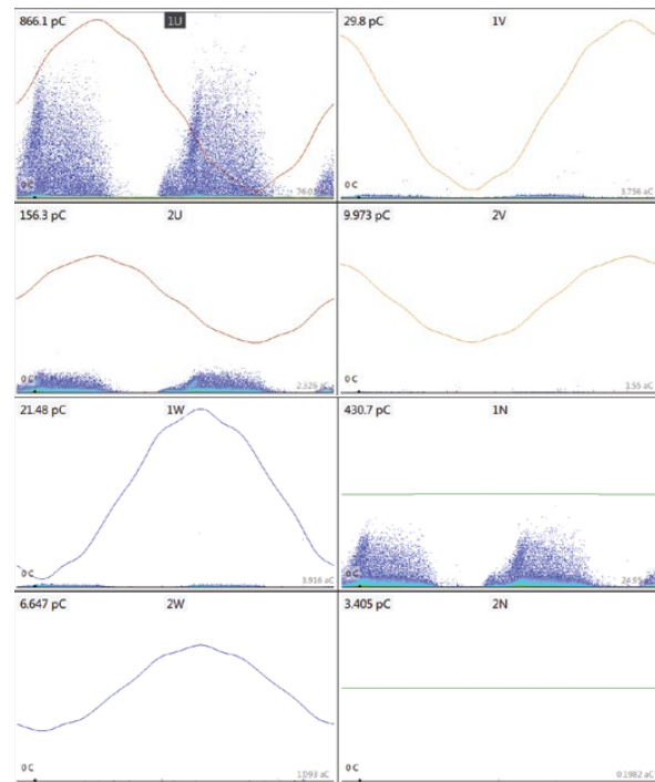
Abbildung 5 An allen Messpunkten bei 0,8 \times U_n ermitteltes PRPD (Phase-Resolved PD)-Muster, lineare Ansicht
