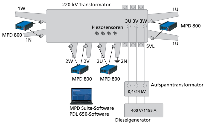
Abbildung 3 Aufbau für die TE-Messungen
