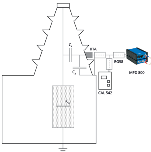
Abbildung 4 Direkt in den Durchführungsmessanschluss eingespeister künstlicher Impuls
