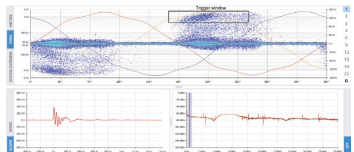
Abbildung 6 MPD Suite-Software; logarithmisch-bipolare Ansicht des PRPD-Musters an 1U, das Trigger-Fenster und das entsprechende Zeit/Frequenz-Signal
