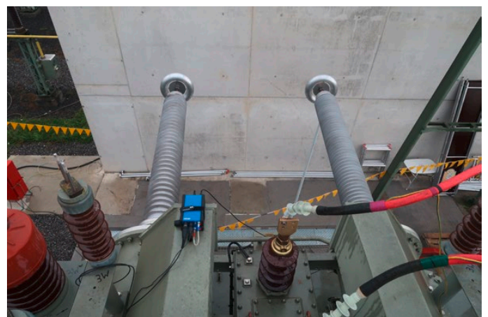
Abbildung 2 Prüfaufbau für TE-Messungen an den Phasen 1U und 1V
