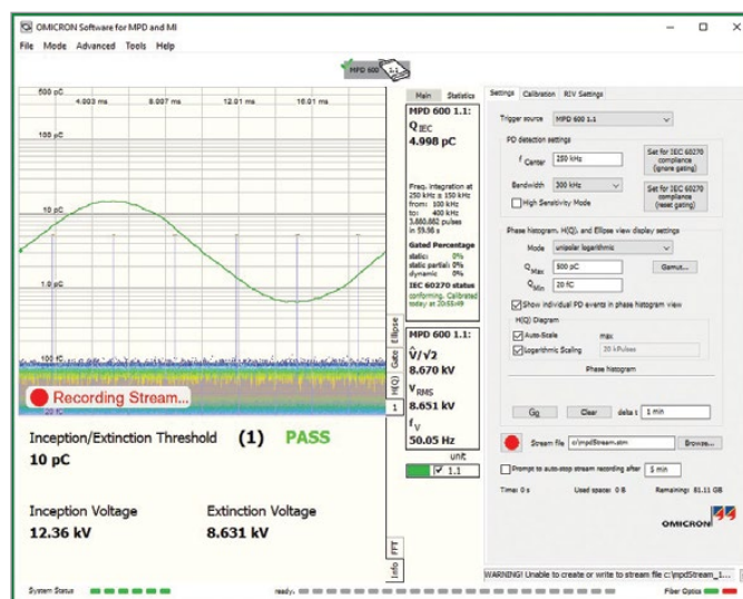
Diagrama PRPD monofásico que muestra la tensión de prueba y el valor de carga, así como la tensión de inicio y extinción (modo básico del MPD 600)
