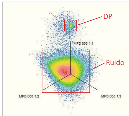
Diagrama trifásico de relación de amplitudes (3PARD)
