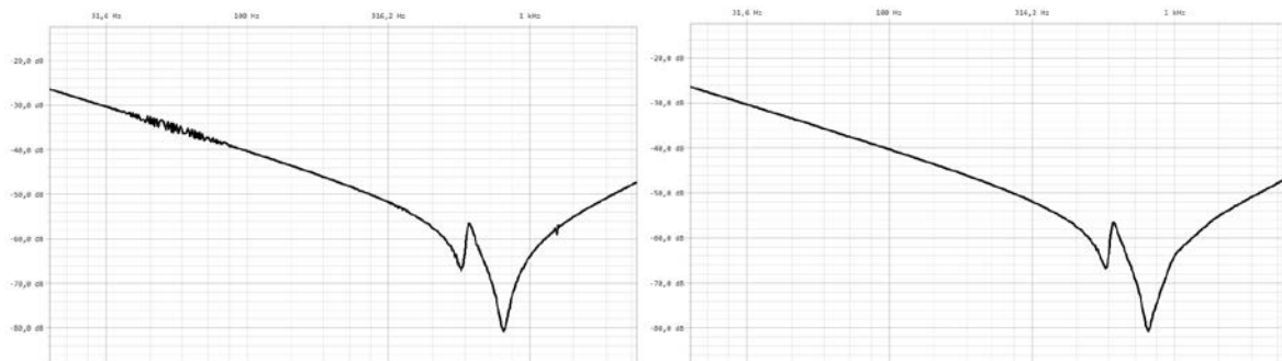
Abbildung 12: Vergleich der SFRA-Kurve links: vor Anwendung von Softwarefilter rechts: nach Anwendung von Softwarefilter.
